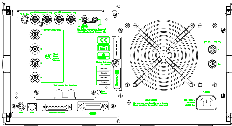
Figure 1-2 4155C/4156C のリア・パネル
